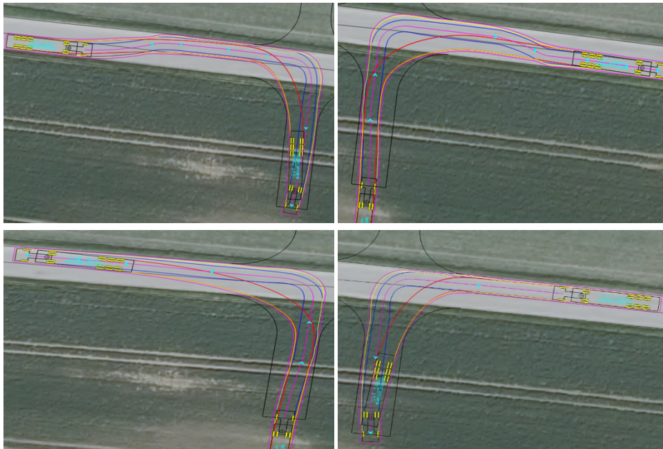
Figur 4: Udsnit fra ansøgning, som viser kørekurver for sættevogntog (SVT) for den sydligere adgang.
