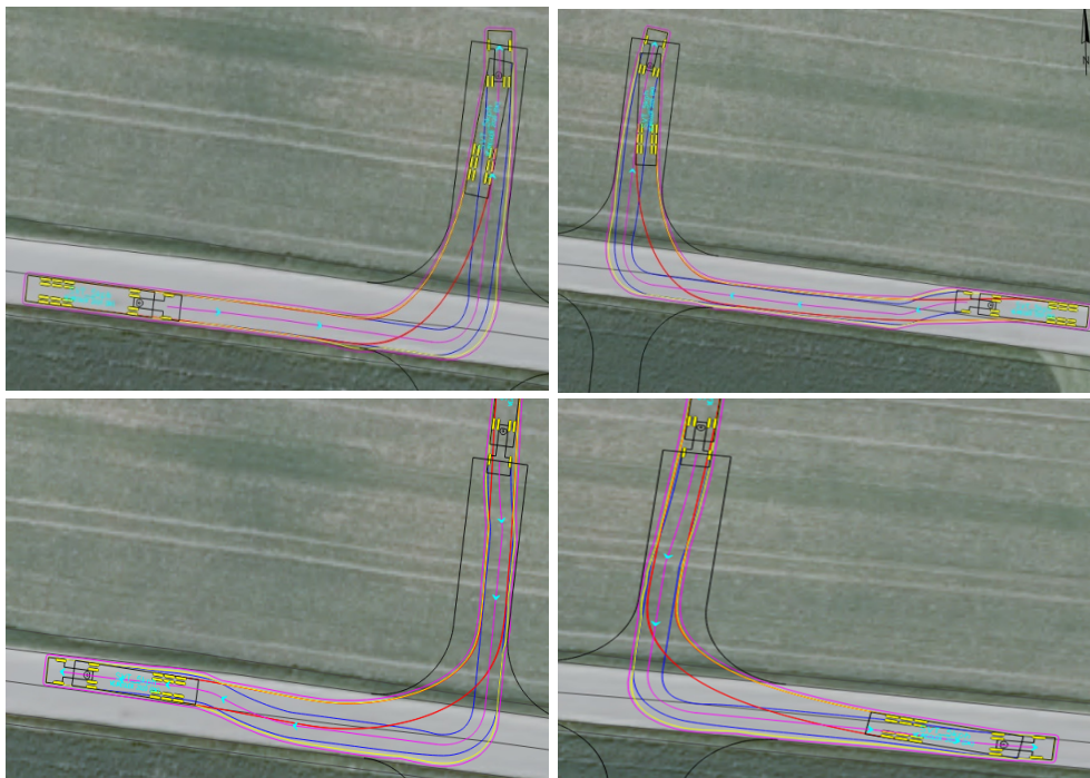
Figur 5: Udsnit fra ansøgning, som viser kørekurver for sættevogntog (SVT) for den nordlige adgang.
