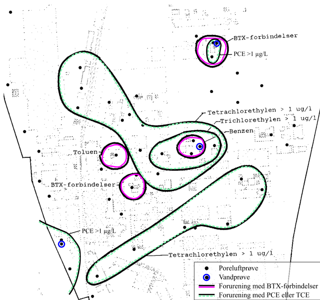
Figur 5: Udbredelse af forurening med benzen, toluen, xylener, PCE og TCE i poreluft på fabriksgrunden i 1990 (efter Krüger, 1992a). Fuldt omrids af fabriksgrunden er vist i figur 3.
