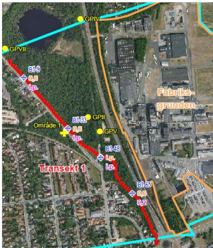
Figur 8: Undersøgelser af poreluft og øvre grundvand nedstrøms for fabriksgrunden (fra COWI A/S, 2011). Røde trekanter: Poreluftmålinger. Blå skrift: Børingsnumre. Orange skrift: Sum af sulfonamider og barbiturater i grundvand ( \mu\text{g/L} ). Pink skrift: Sum af chlorerede opløsningsmidler ( \mu\text{g/L} ). Bemærk: GPII er placeret for langt mod nord og GPV er placeret for langt mod vest, da den reelt står umiddelbart øst for Simmelbrovej. Se figur 1.
