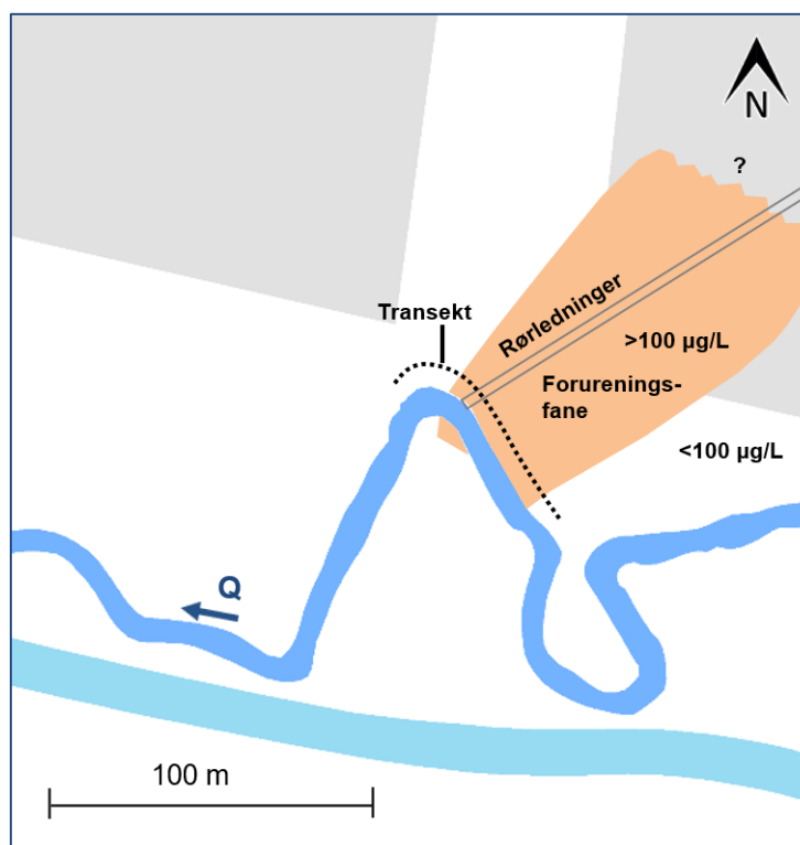
Figur 13: Hotspot for udsivning af forurening til Grindsted Å (efter Rønde, 2019). Placeringen af udsnittet er vist på figur 1.
