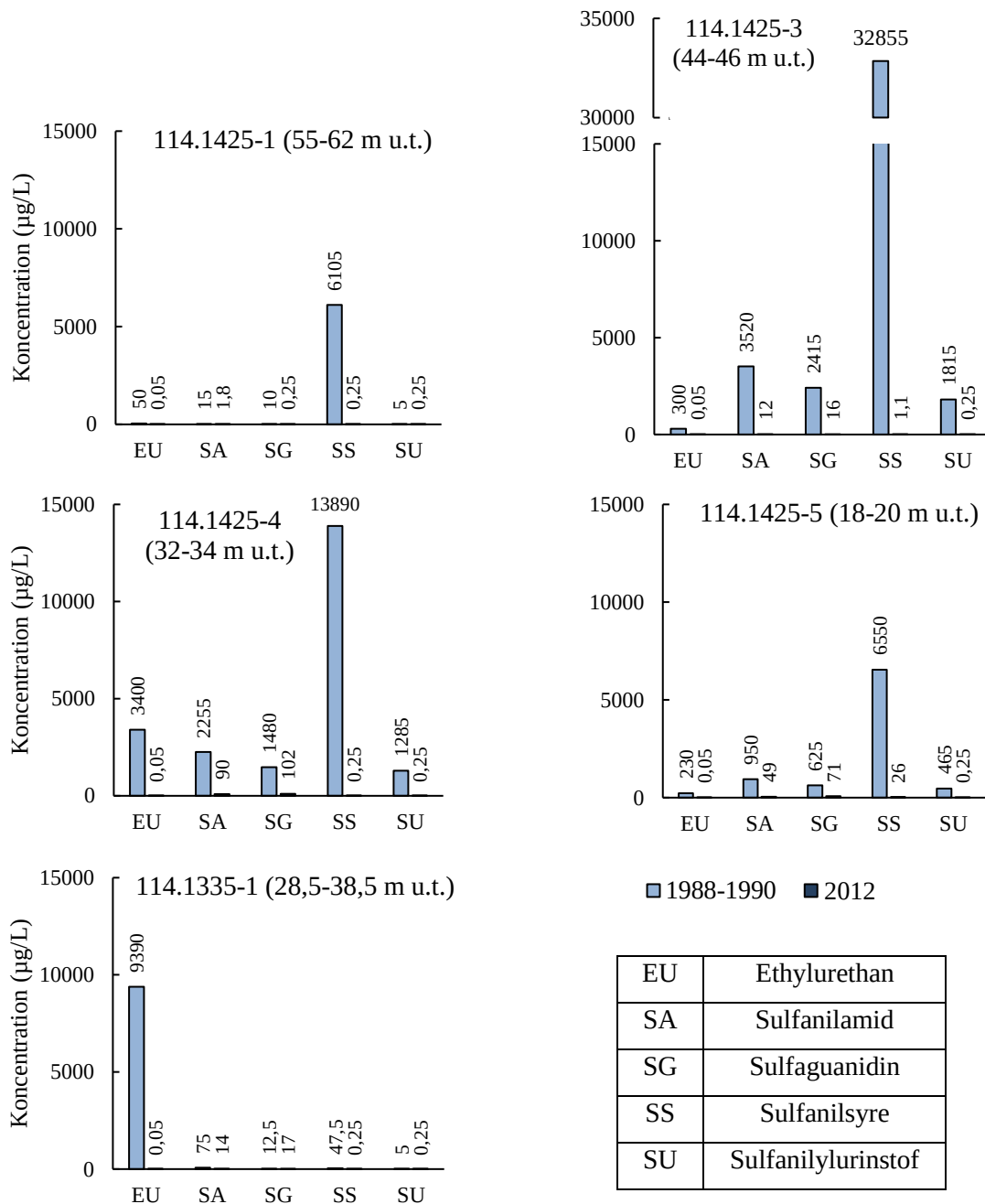
Figur 6: Grundvandskoncentrationer af fem farmaceutiske stoffer i borer umiddelbart nedstrøms for Grindstedværkets tidligere grund. Der sammenlignes mellem perioderne 1988-1990 (lyseblå) og 2012 (mørkeblå). Tallene over stavene angiver koncentrationerne i µg/L.
