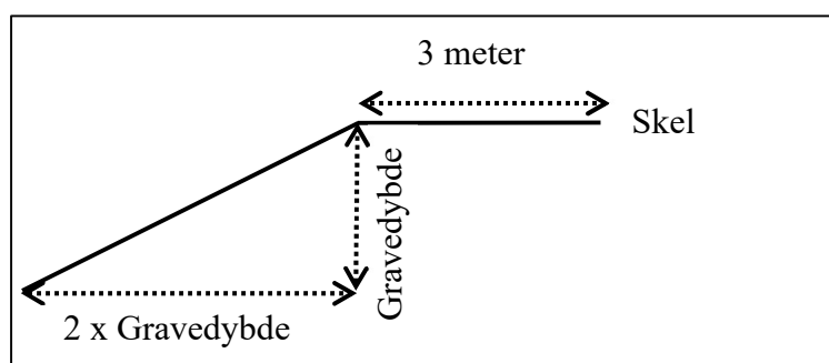
Principskitse for gravning nær privat vej, digefod til beskyttede diger og naboskel.
